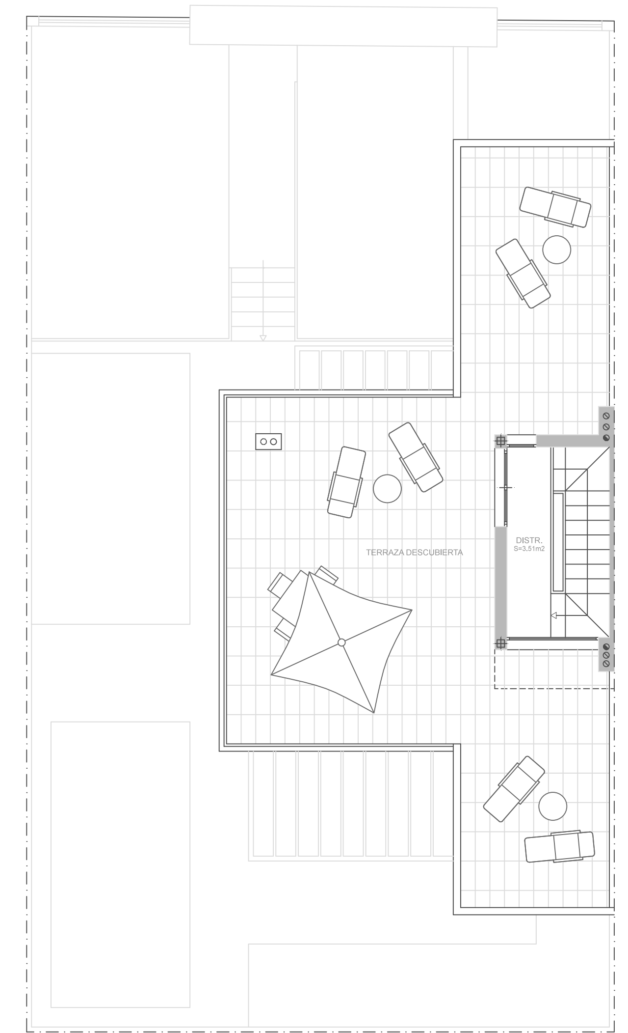
PLANTA TORRE
